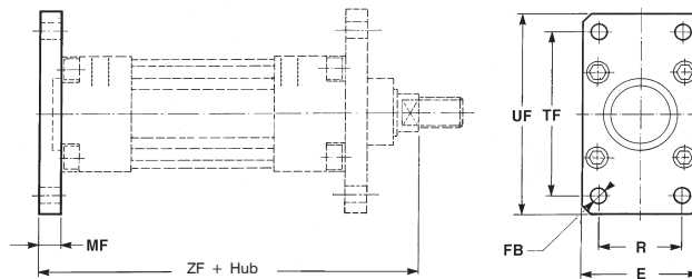
Hintere Montage
