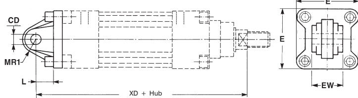
Hinteres Gelenklager
