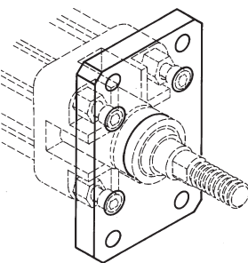
Gelenkabmessungen ISO MP2 - MP4
