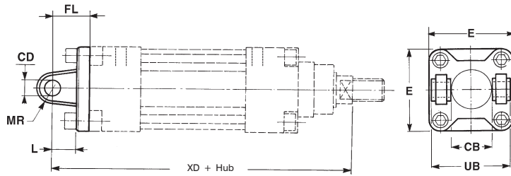
Hinterer Gelenklagerbock
