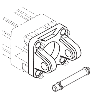
Hinterer Gelenklagerbock
